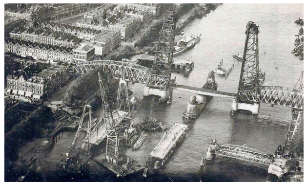
De Hef in Rotterdam 1926
