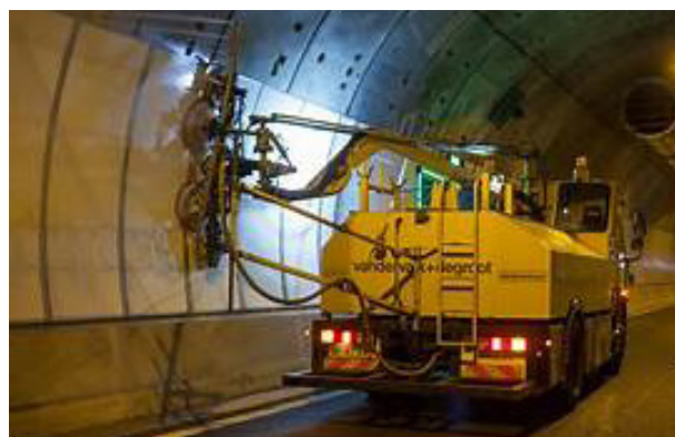
Bouw Westerscheldetunnel
